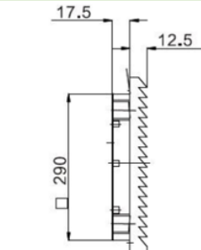
侧视图(出口) Side View (Outlet)
