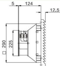
侧视图(入口) Side View(Inlet)
