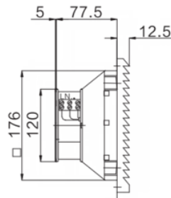
侧视图(入口) Side View(Inlet)
